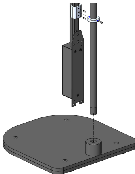
б) монтаж на штативе
