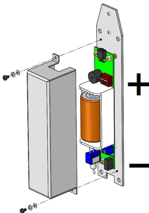
Рисунок 2.1 - Установка элементов питания в блок извещателя
