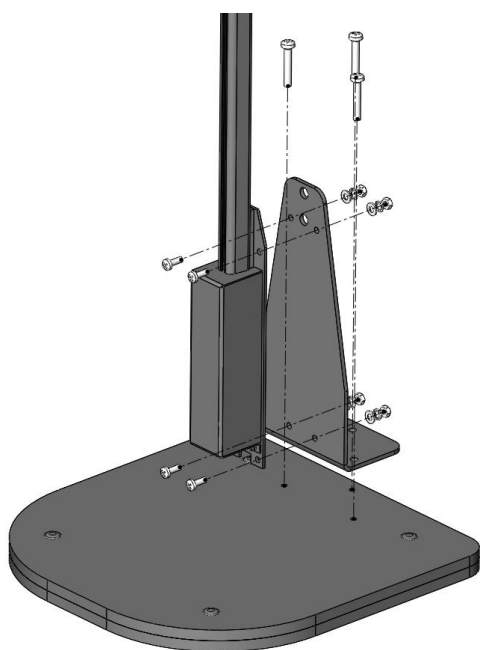
а) монтаж на постаменте
